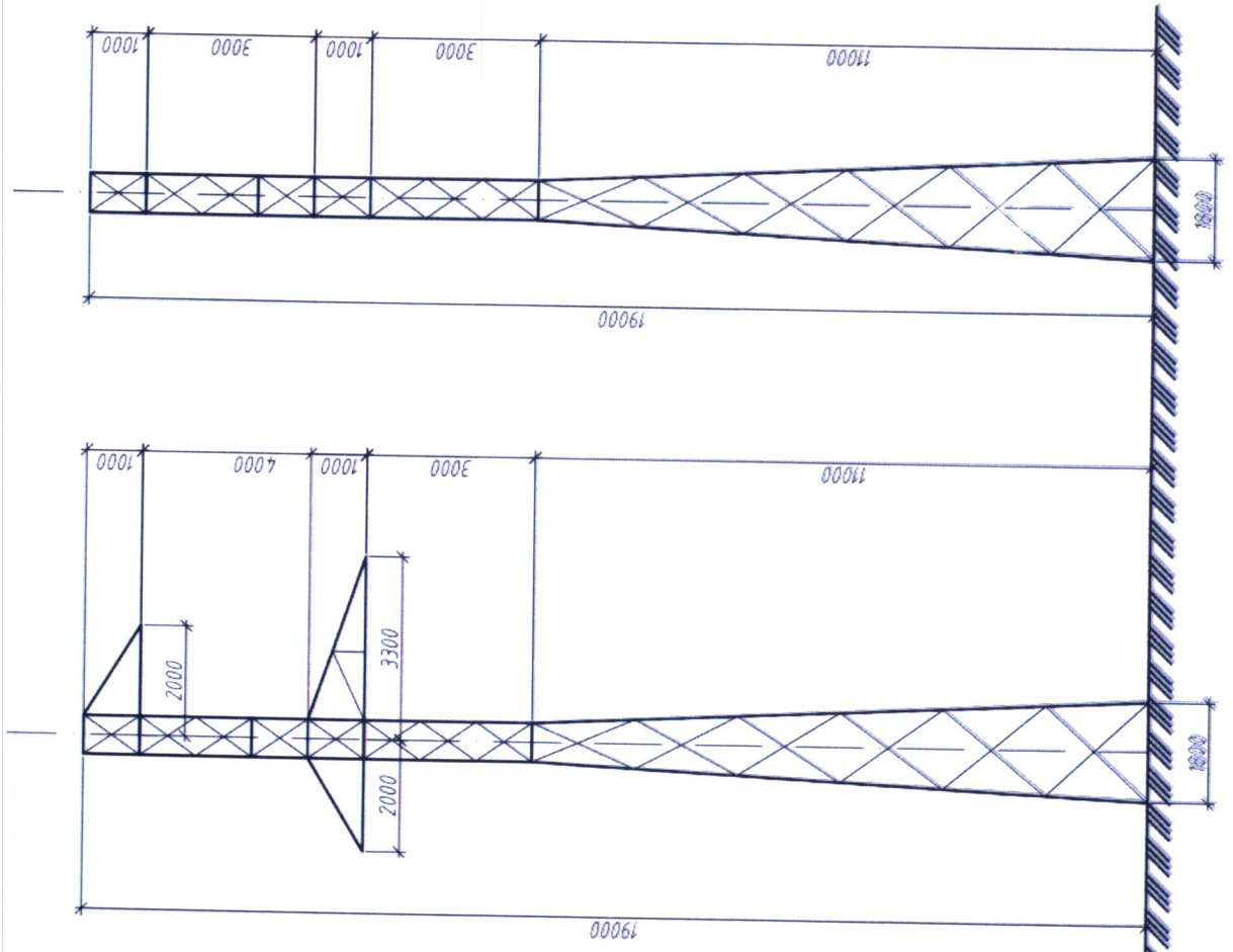
Вариант опоры П35-1 для III - IV районов по гололеду
