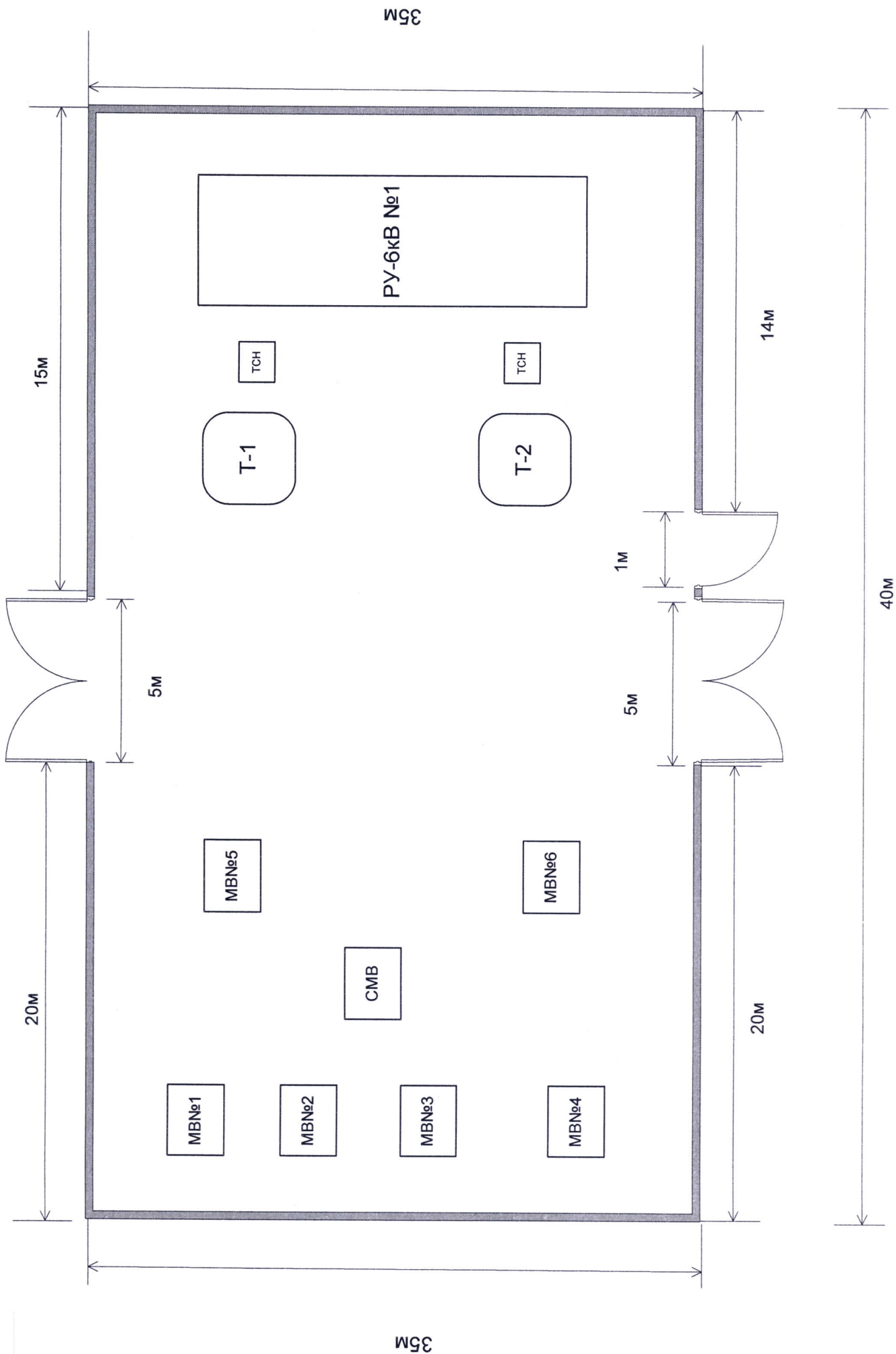
План – схема ограждения ПС 35/6кВ КНС-4
